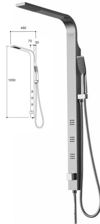
Colonna doccia multifunzione in acciaio inox con trattamento antimpronta e sistema anticalcare, soffione doccia superiore con effetto pioggia N° 3 body jet, deviatore, doccia estraibile, adatto per installazione a parete abbinabile ad un incasso doccia o esterno doccia
