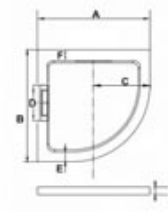
Piatto Doccia R=55
