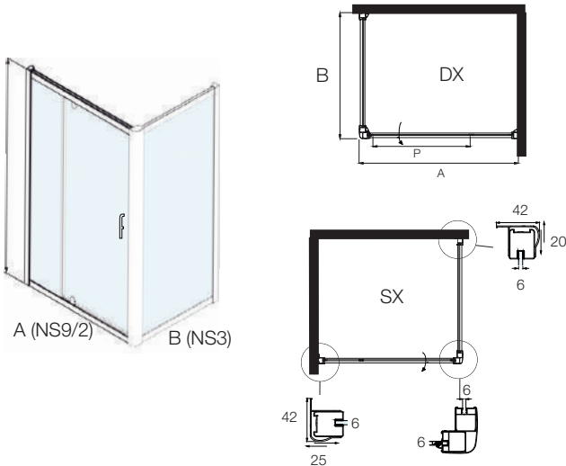
Laterale fisso NS3-19 in abbinamento alla porta a battente NS9
